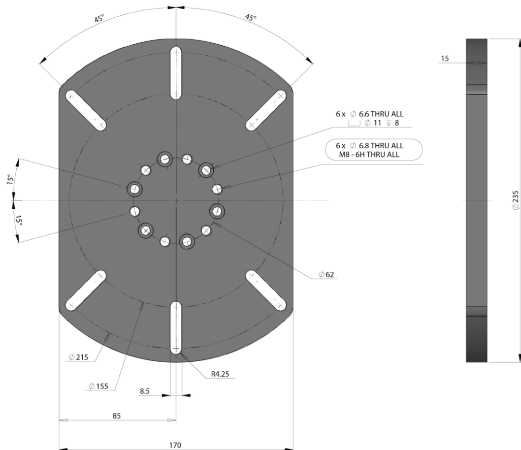
Fig. 46 : Base plate dimensions
