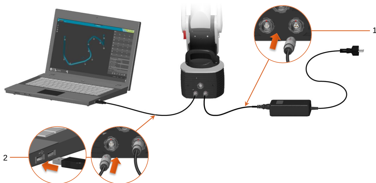
Fig. 31 : USB connection
