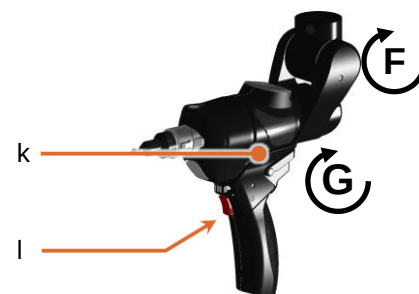
Fig. 10 : 7-axes Wrist
